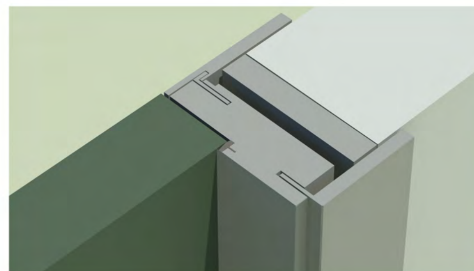
Sezione porta a battente versione "plana"
