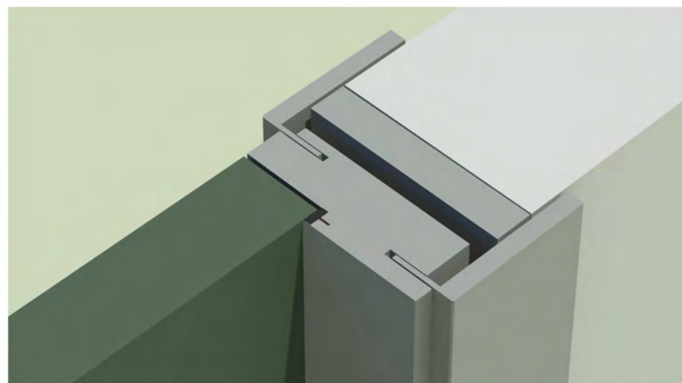
Sezione porta a battente con cerniere a scomparsa
