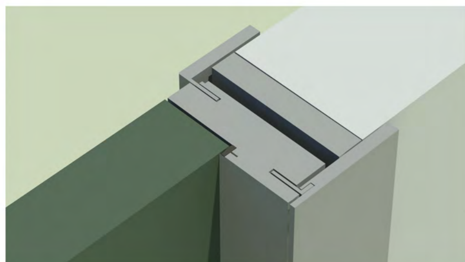
Sezione porta a battente con coprifilo esterno da 10 cm
