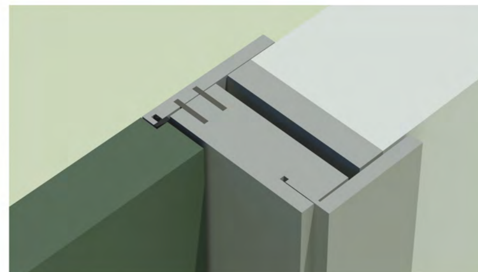
Sezione porta coplanare con apertura inversa
