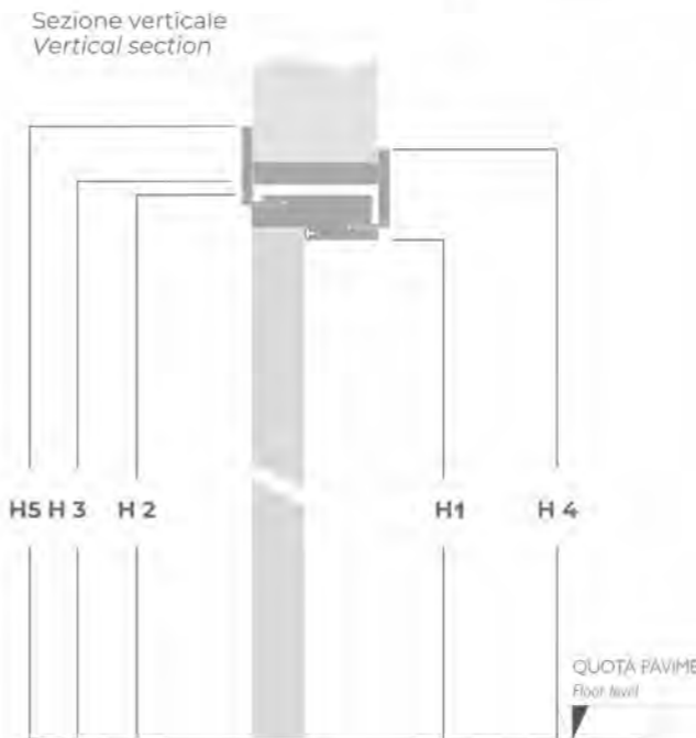
Apertura Destra Right opening
